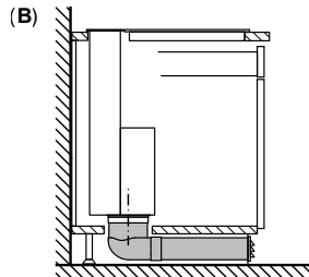
B: Buitenwand – U-waarde > 0,5 W/(m²K)
