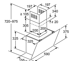
Afmeting in mm Apparaat in luchtcirculatiemodus
