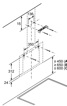
Wandinstallatie met luchtkanaal
